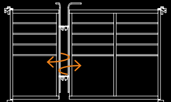
Apertura total por cierre tipo varilla. (accionamiento desde pasarela)
