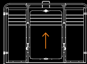
Apertura manual de 1450 mm. (accionamiento desde pasarela)
